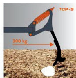
Rugóerő - talajellenállás TOP-S és SPEC HD esetén
